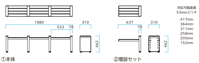
①本体 245-0100 (組立例) 組立例：座高/417mm・311mm・205mm
